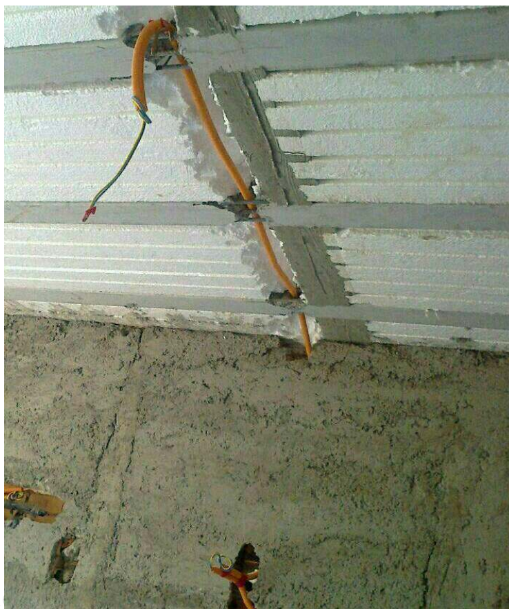
نمونه‌ای از سیم کشی توکار (از سقف و دیوار)
