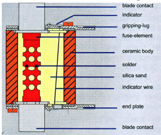
شکل ۴،۱- فیوز مدل NH
