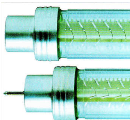
شکل ۴،۵- فیوزهای Full Range - بالا: نو - پایین: عمل کرده
