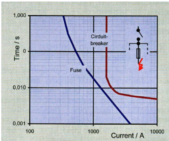
شکل ۲،۷- کلید بالادست فیوز
