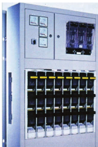
شکل ۳-۱۴ - تابلوی توزیع با کلید فیوز عمودی
