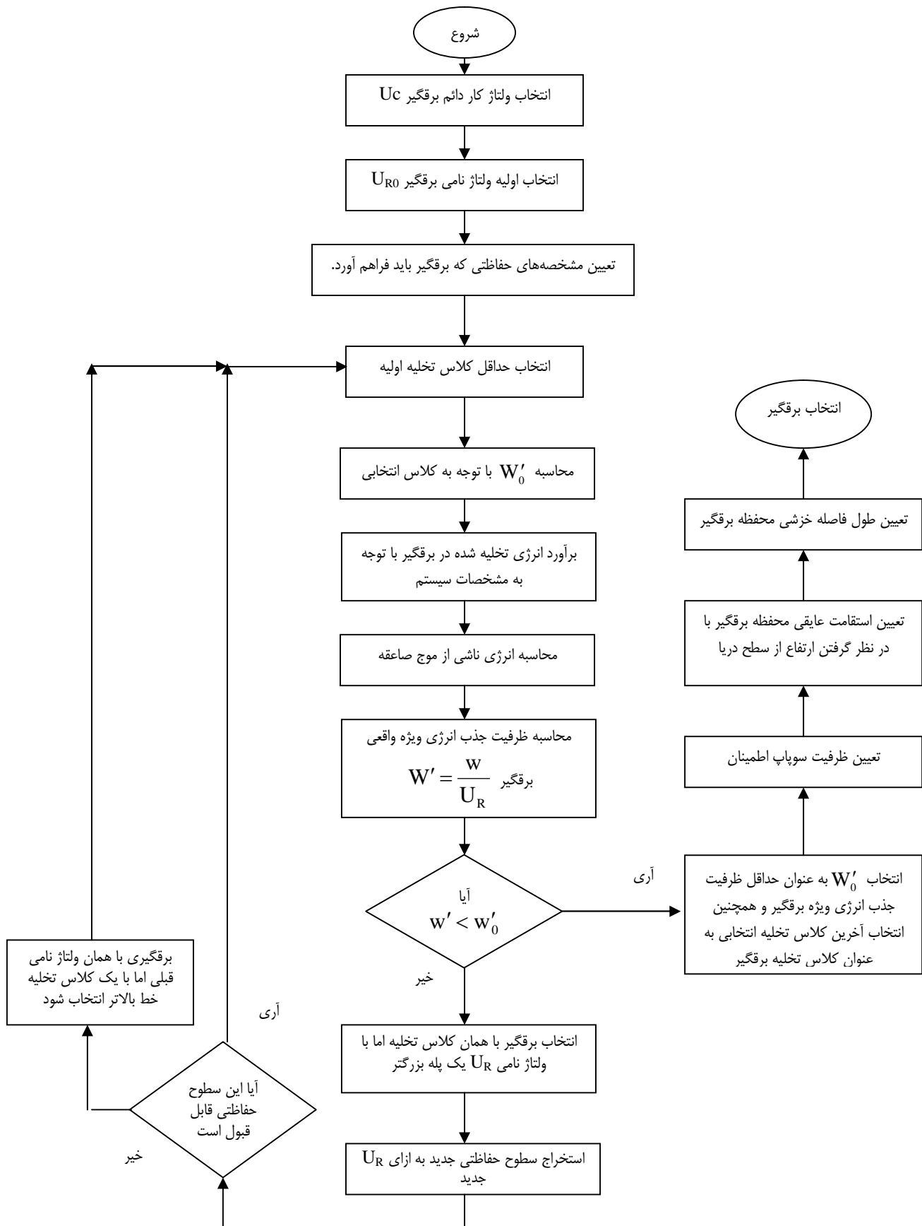
شکل ۲-۱: رویه گام به گام انتخاب پارامترهای برقی
