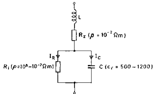
شکل ۳-۱: مدار معادل دیسکهای اکسید فلز بر فکیر
