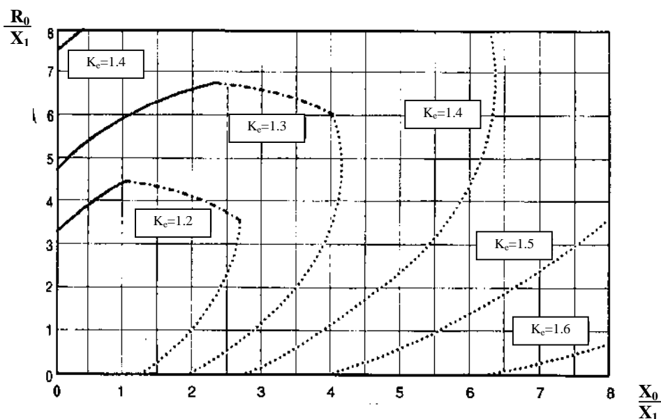
شکل ۲-۱۵: نسبت بین R_0/X_1 و X_0/X_1 برای مقادیر ثابتی از ضریب اتصال زمین که در آن R_1=2 X_1 است
