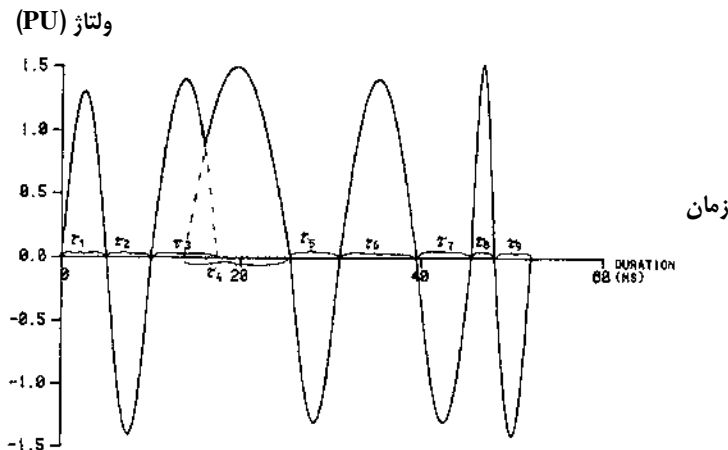
شکل ۲-۱۶: مثالی از TOV متشکل از چندین فرکانس مختلف متفاوت از فرکانس قدرت
