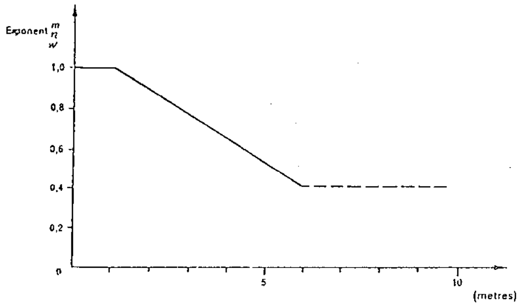
شکل ۲-۱۸: ضرایب n, m و w برای الکترودهای جدول (۲-۱۱) برحسب فاصله بین الکترودها
