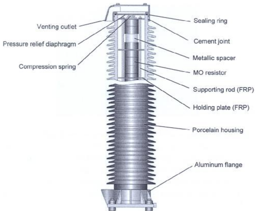
شکل ۲-۲۱: برش شماتیکی از برقیگیر
