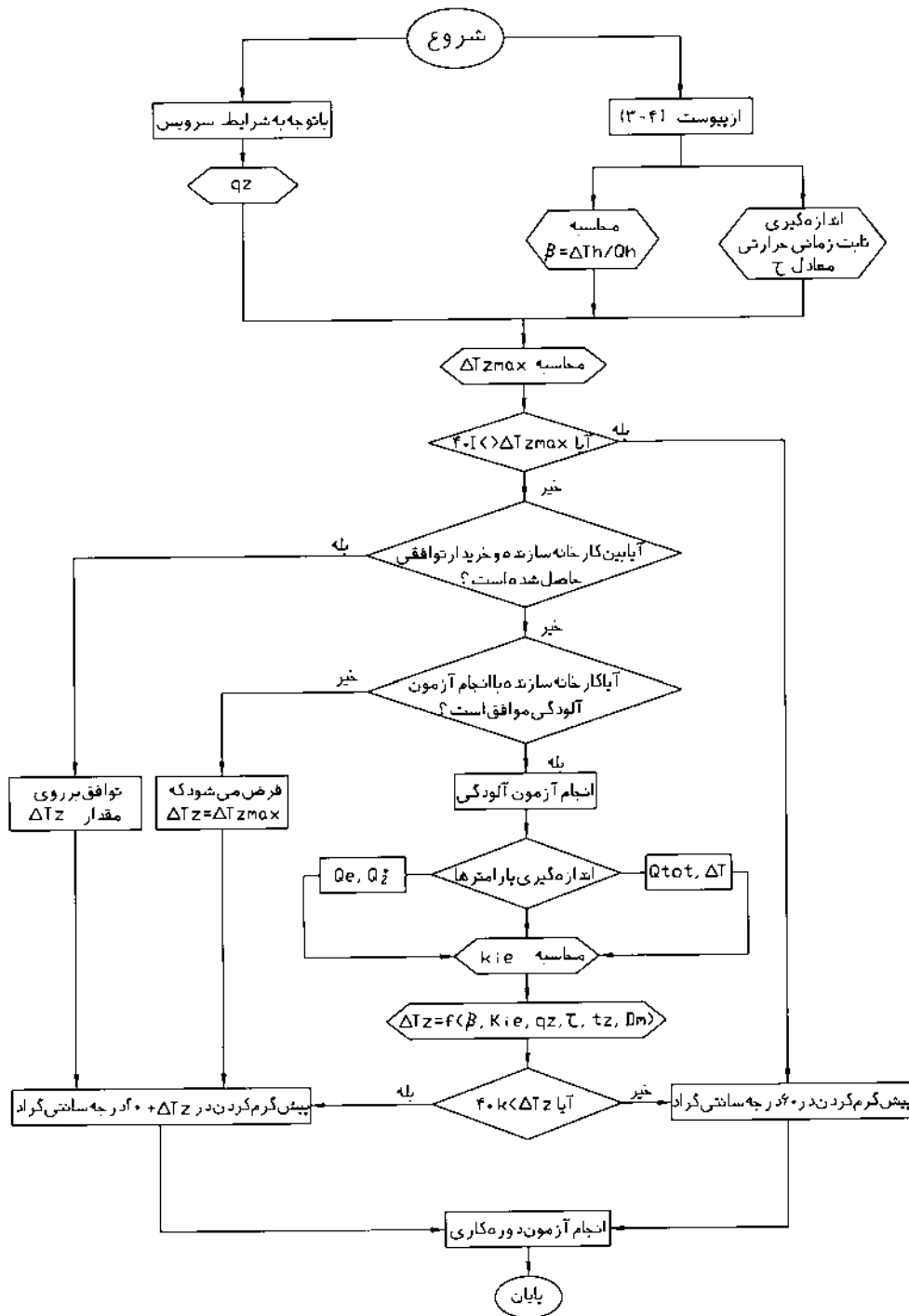
شکل ۳-۲: فلوجارت تعیین دمای شروع آزمون دوره کاری
