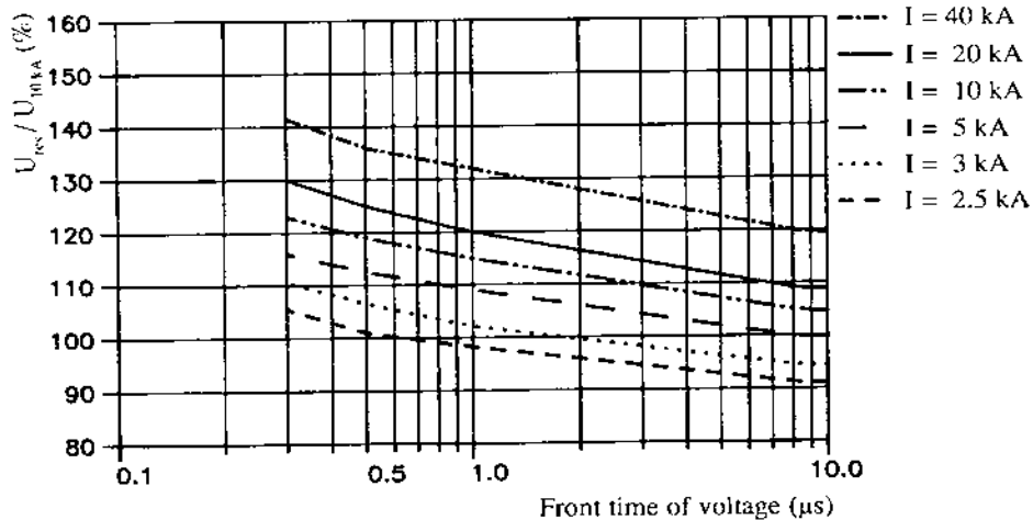
شکل ۲-۷: تغییر ولتاژ تخلیه برقگیر در اثر تغییر زمان پیشانی موج جریان صاعقه
