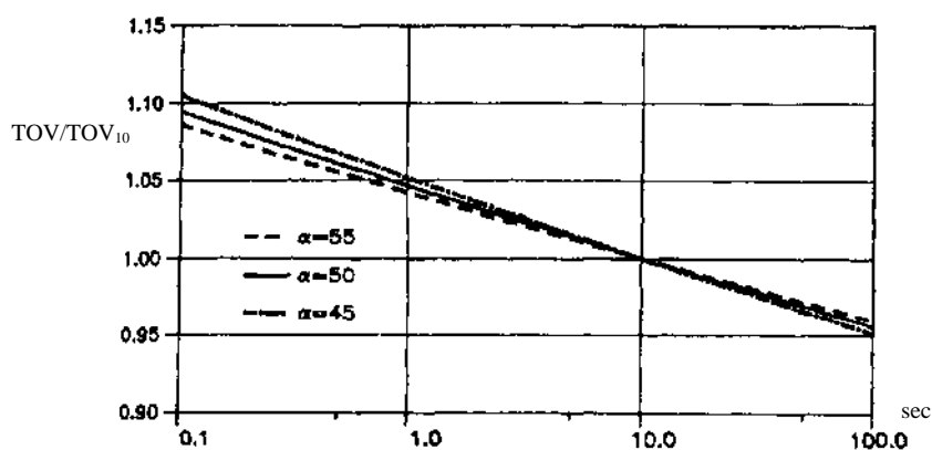
شکل ۳-۲: منحنی قابلیت TOV بر حسب زمان برای یک برقی با \alpha های متفاوت
