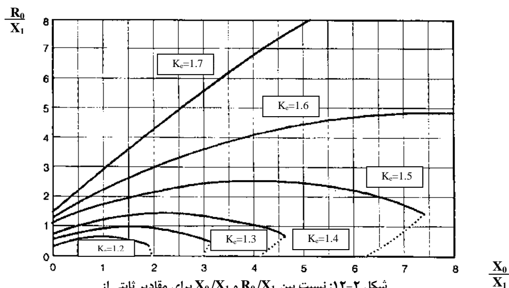
شکل ۲-۱۲: نسبت بین R_0/X_1 و X_0/X_1 برای مقادیر ثابتی از
