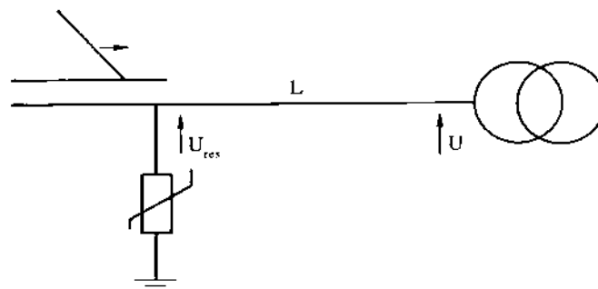
شکل ۲-۵: دیاگرام ساده‌ای جهت ارزیابی اثر فاصله برقگیر از موضع تحت حفاظت
